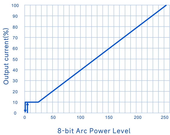
线性调光曲线:(DMX机型)
